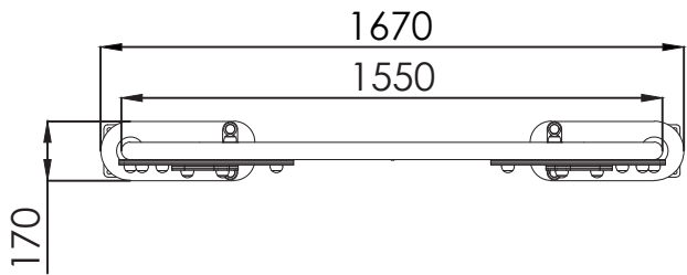
PLANTA
