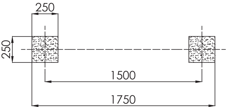
CIMENTACIÓN
