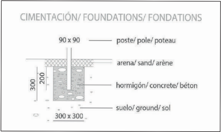
CIMENTACIÓN
