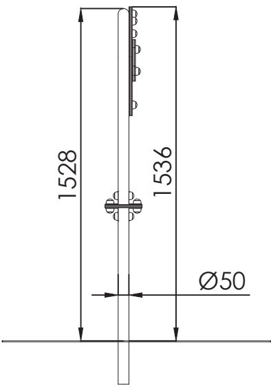
PERFIL
