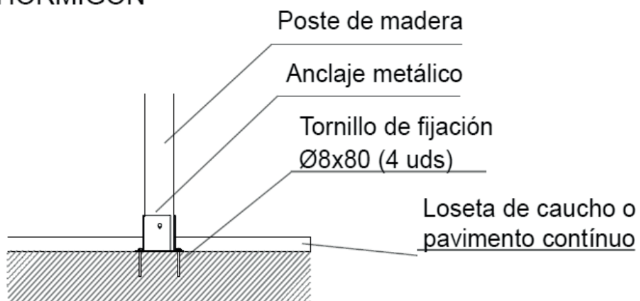
ESQUEMA DE CIMENTACIÓN EN HORMIGÓN
