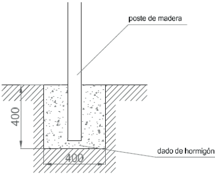
DETALLE DE CIMENTACIÓN
