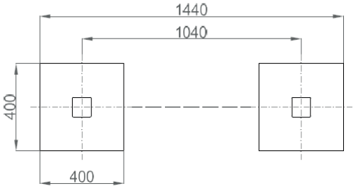
PLANTA CIMENTACIÓN
