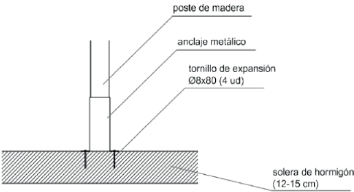
DETALLE DE ANCLAJE
