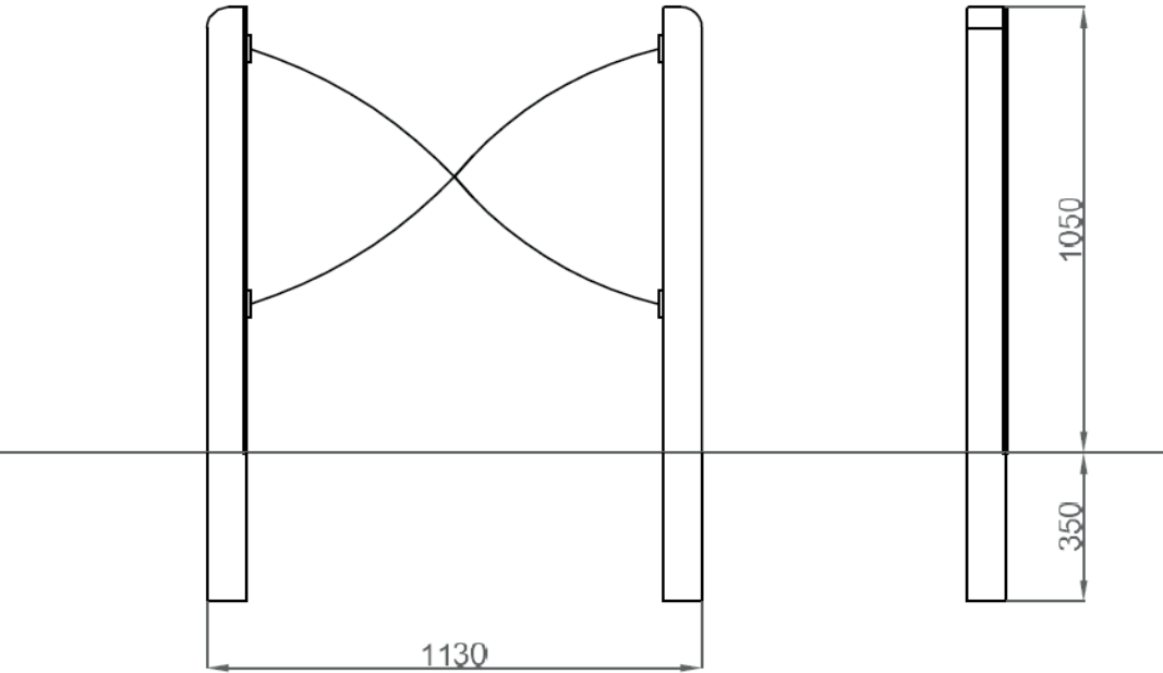
ALZADO
