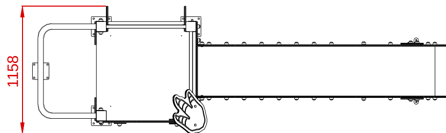
PLANTA
