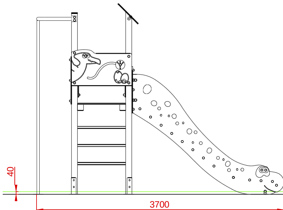
ALZADO
