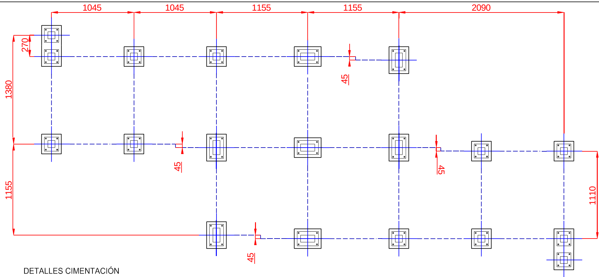
ESQUEMA DE CIMENTACIÓN EN ARENA
