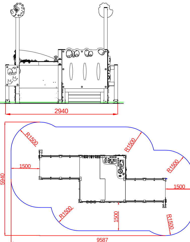
PERFIL IZQUIERDO
