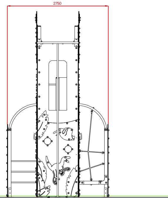
PERFIL
