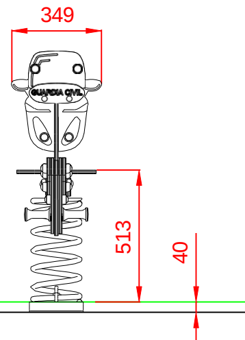
PERFIL
