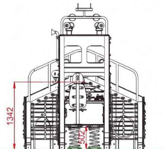
PERFIL DERECHO
