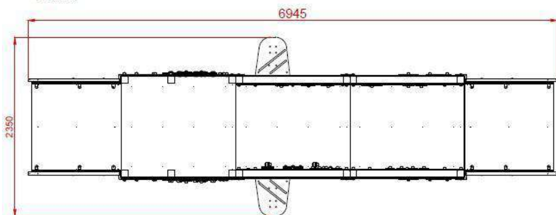
PLANTA
