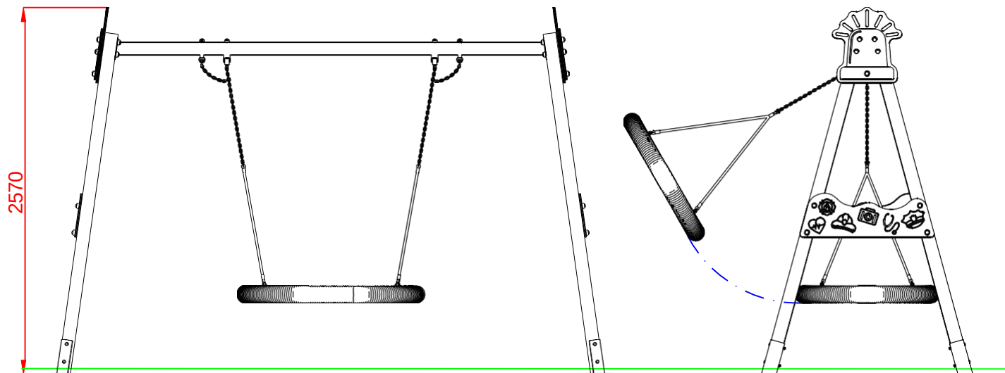
ALZADO
