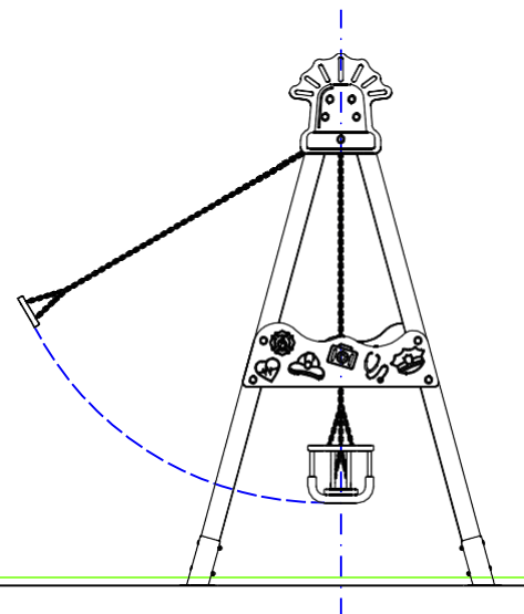
PERFIL IZQUIERDO
