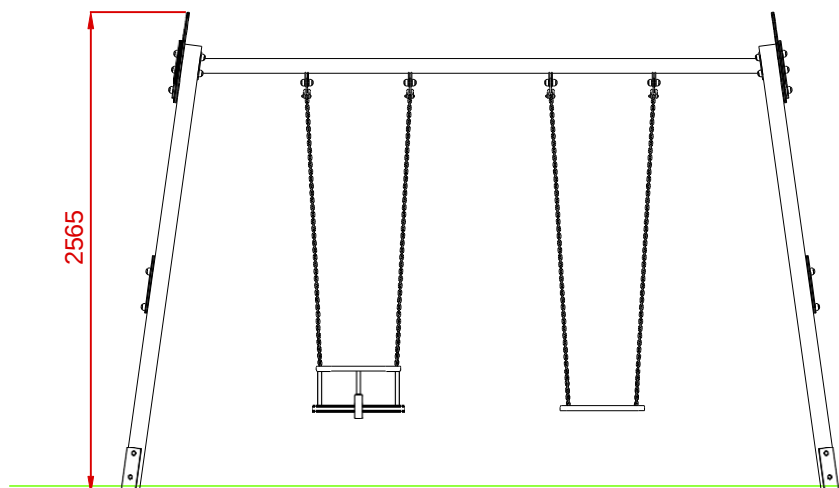
ALZADO
