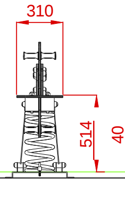
PERFIL
