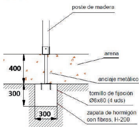
ESQUEMA DE CIMENTACIÓN EN ARENA
