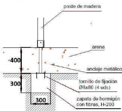
ESQUEMA DE CIMENTACIÓN EN ARENA
