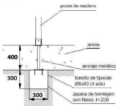
ESQUEMA DE CIMENTACIÓN EN ARENA
