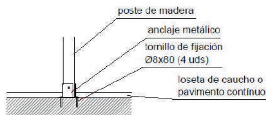
ESQUEMA DE CIMENTACIÓN EN HORMIGÓN
