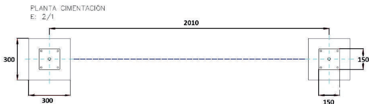
ESQUEMA DE CIMENTACIÓN EN ARENA
