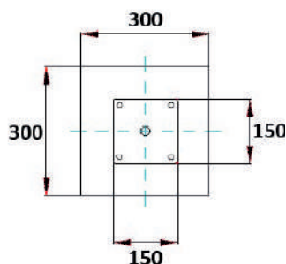
PLANTA CIMENTACIÓN E: 2/1
