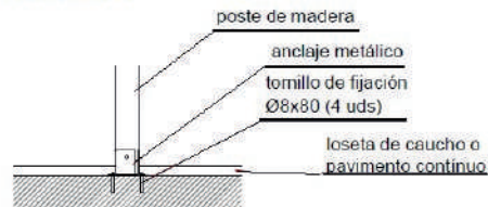
ESQUEMA DE CIMENTACIÓN EN HORMIGÓN
