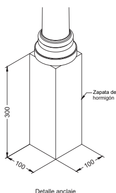
Detalle anclaje
