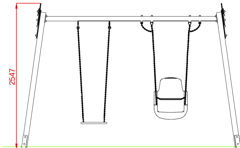
ALZADO
