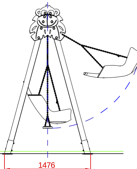
PERFIL IZQUIERDO
