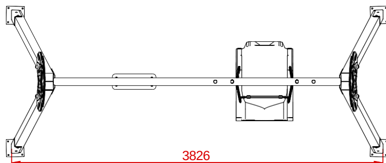
PLANTA
