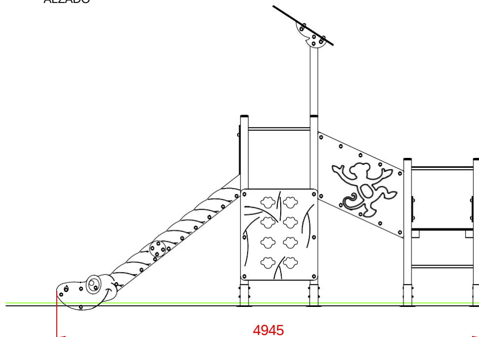
ALZADO
