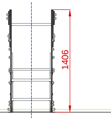
PERFIL IZQUIERDO
