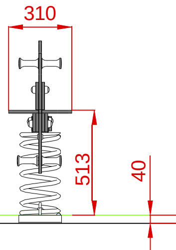
PERFIL
