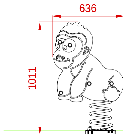
ALZADO
