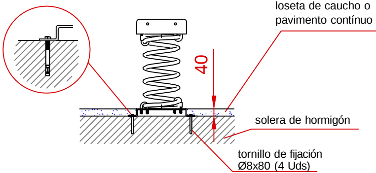
Detalle de sujeción de espirro metálico
