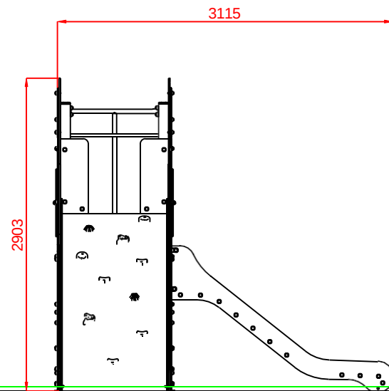
PERFIL IZQUIERDO
