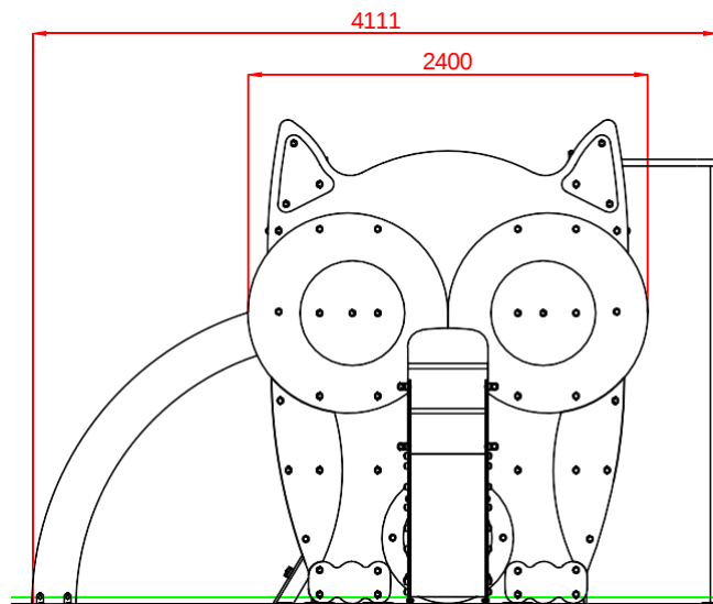
ALZADO
