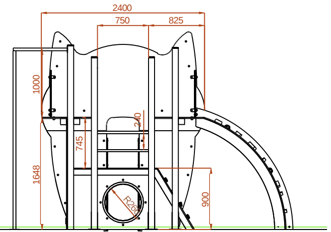
ALZADO POSTERIOR SECCIONADO
