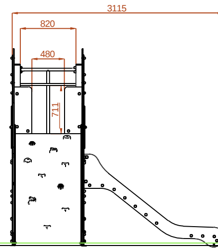
PERFIL IZQUIERDO
