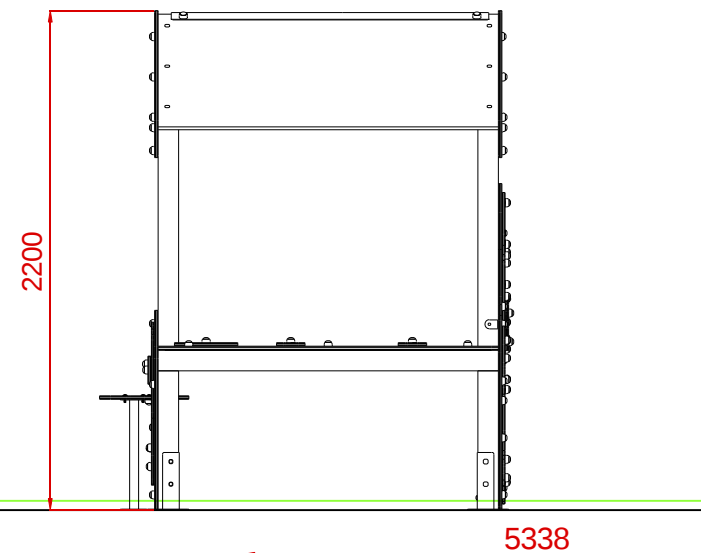
PERFIL
