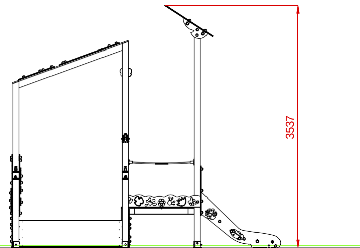
PERFIL IZQUIERDO
