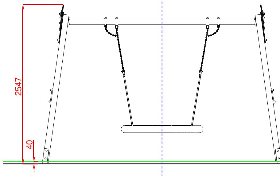
ALZADO
